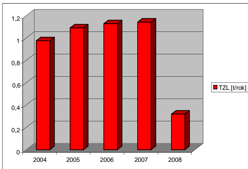
Obr. 11 Vývoj emisií TZL prevádzkovateľa Slovokord
