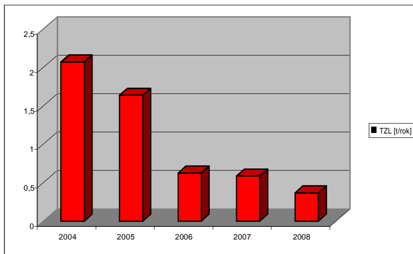
Obr. 10 Vývoj emisií TZL prevádzkovateľa Kordservice
